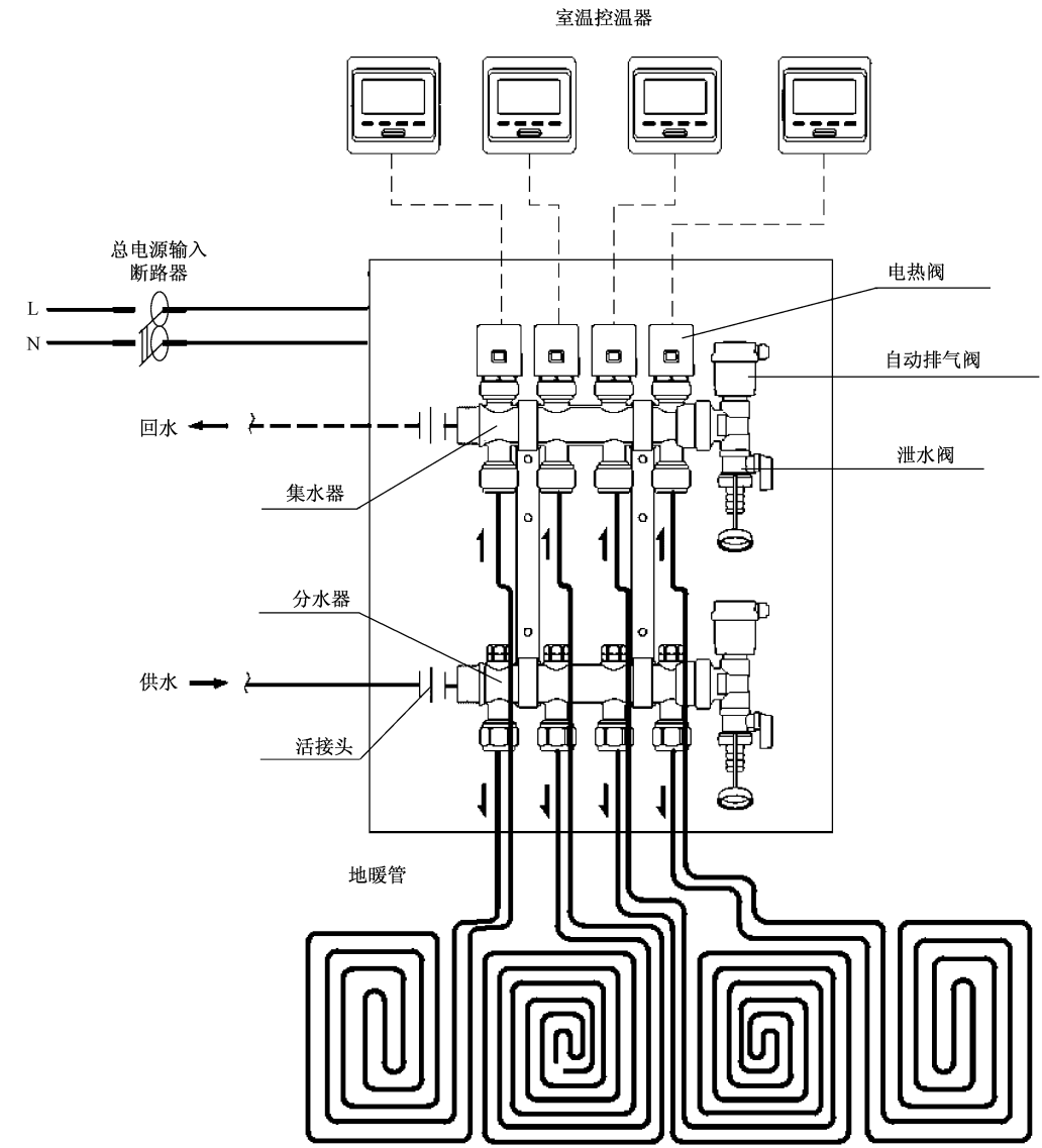
图 A.4 水地暖分室控温系统中控温器接线图
